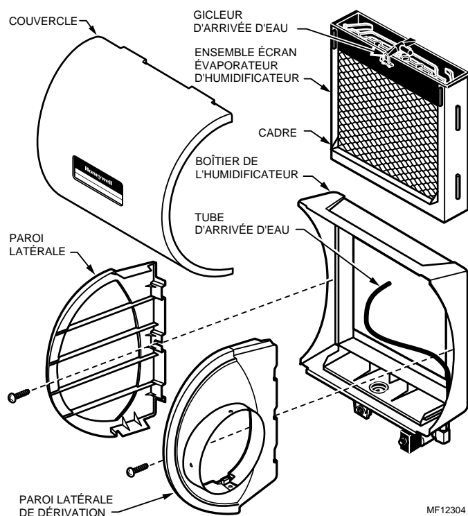
Fig. 2. Composants de l'humidificateur.
